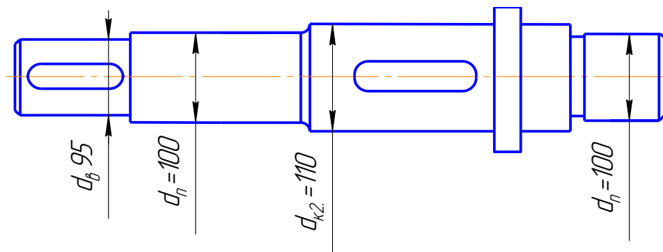
Рис. 37. Вал редуктора
