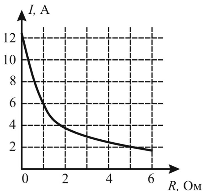
Рис. 6.4. Зависимость силы тока от сопротивления.
