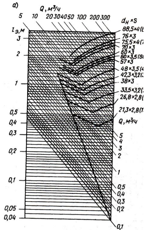
Рисунок 2.2 - Номограмма для определения эквивалентных длин
