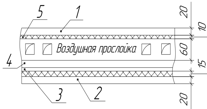
Рисунок 3 - Бесчердачное перекрытие. Потолок.
