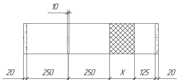
Рисунок 1 - Наружная стена
