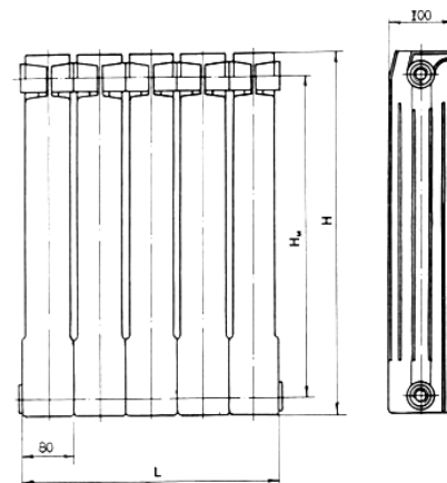
Рисунок 5 - Габаритные размеры радиатора «Сантехпром БМ»
