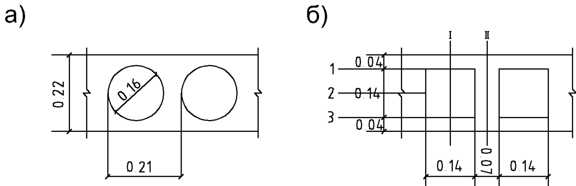
Рисунок 2 - Многопустотная бетонная плита
