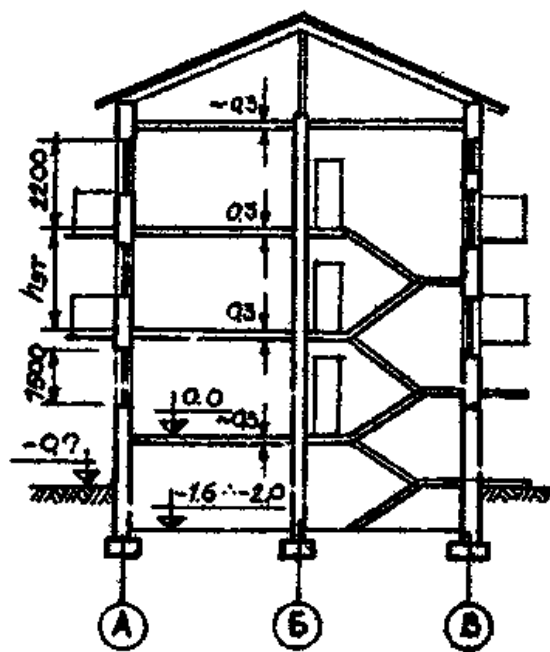
Рисунок 1 – Профиль жилого трехэтажного здания
