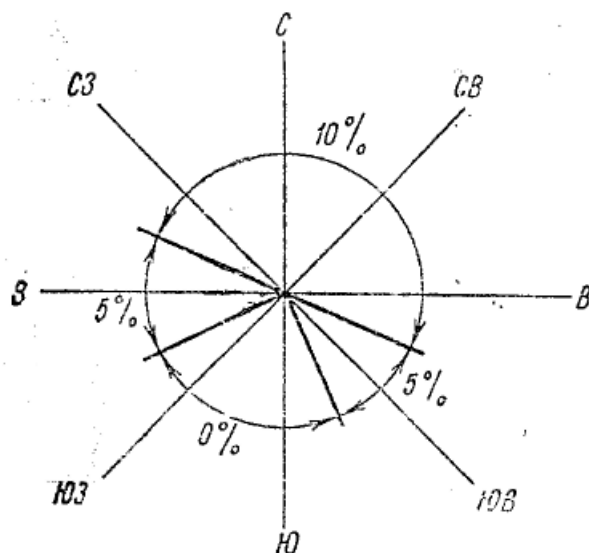
Рисунок 4 - Величины добавок к основным теплопотерям в зависимости от ориентации ограждения по странам света
