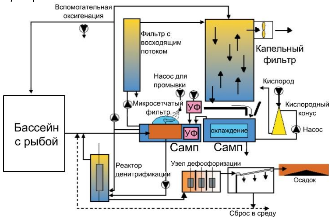
Рисунок 1- Схема УЗВ
