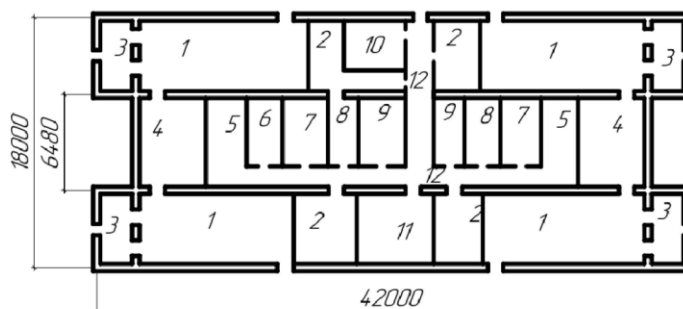
Экспликация помещений
