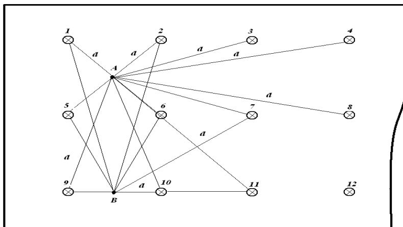
Рис.5. Фрагмент помещения с нанесенными контрольными точками.
