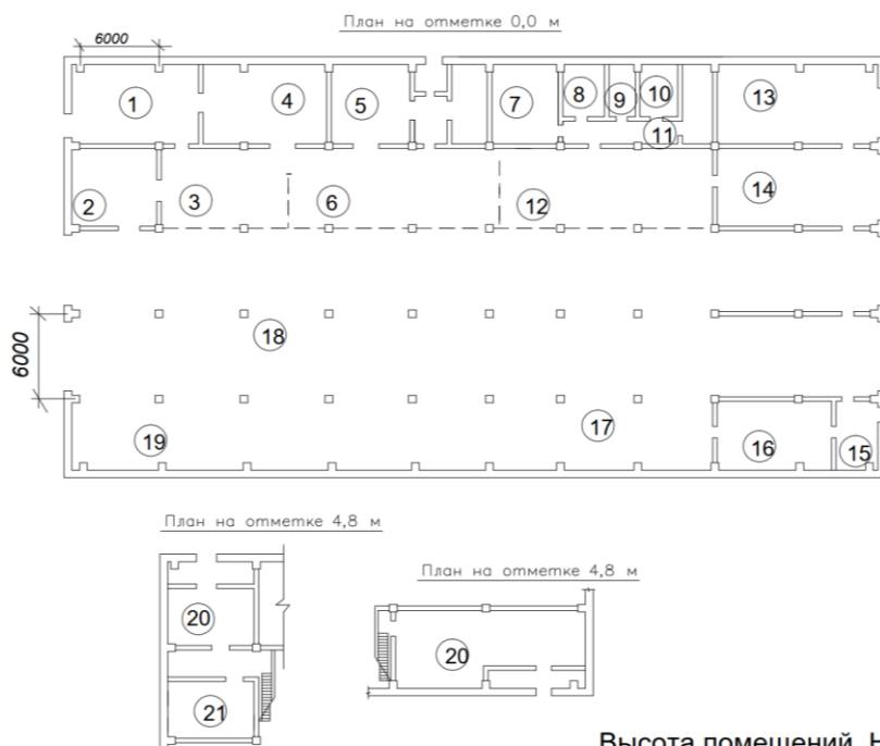
Экспликация помещений
