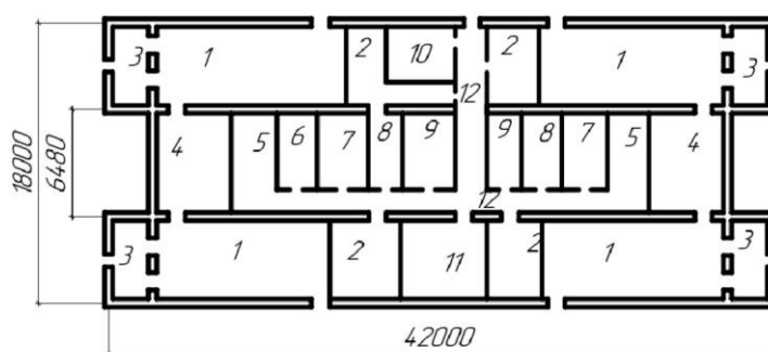
Экспликация помещений
