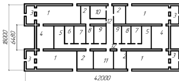
Экспликация помещений
