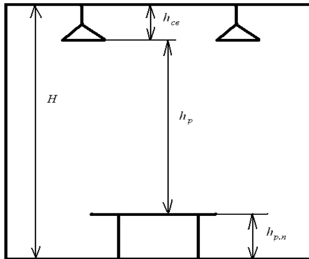
Рис.1. Определение расчетной высоты.
