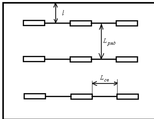
Рис.3. Расположение светильников с люминесцентными лампами.
