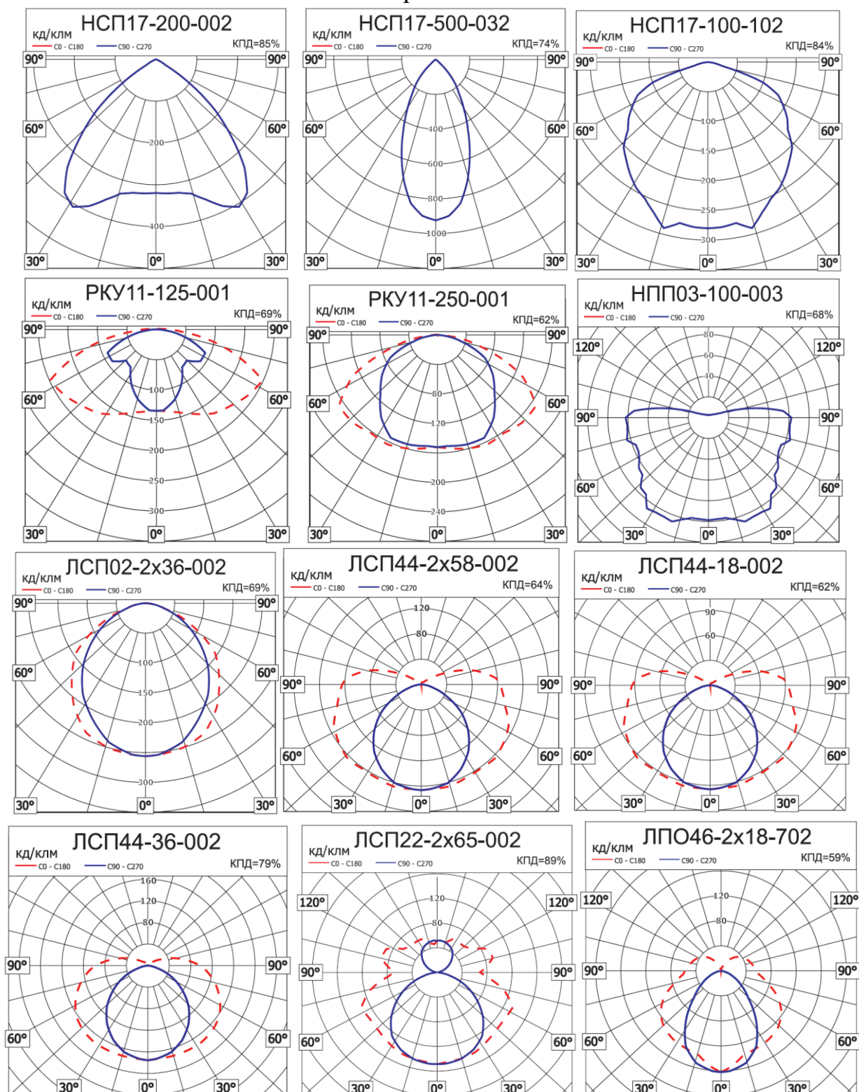
Рис. 7. Кривые силы света в абсолютных единицах при световом потоке источника света равном 1000 лм.
