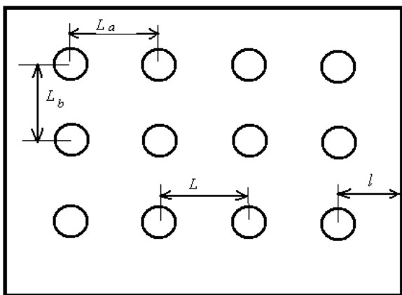
Рис.2. Расположение светильников с лампами накаливания.
