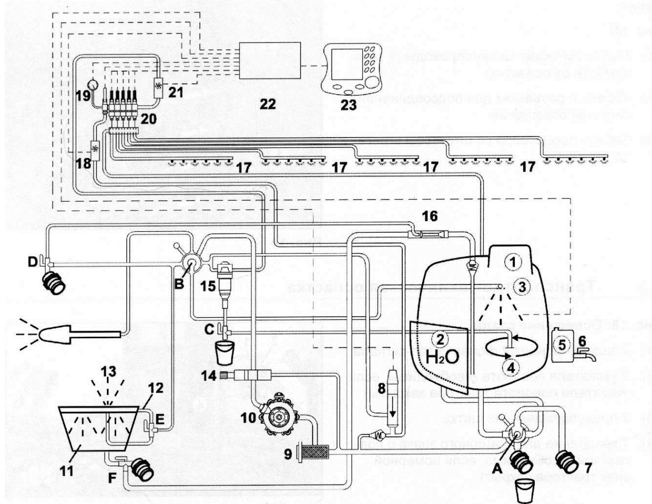
Рис. 32. Технологическая схема работы опрыскивателя UF-1501
