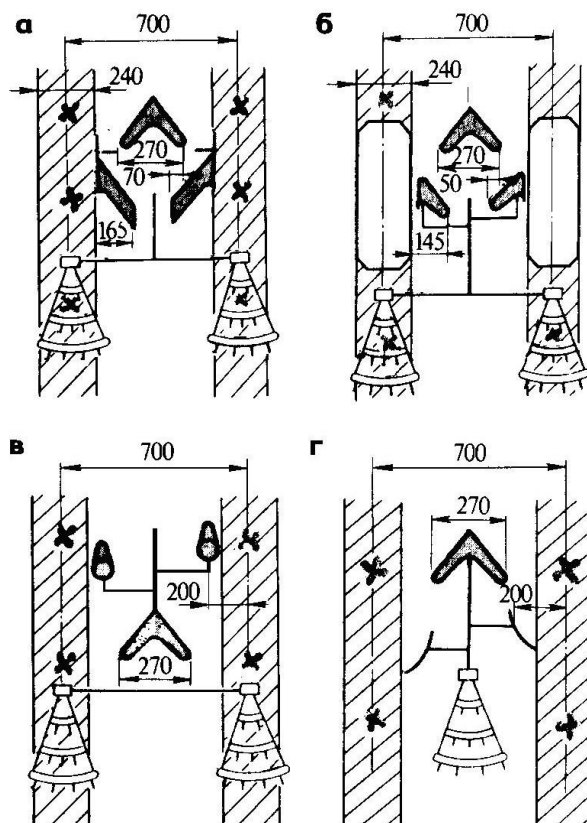
Рис. 12. Схемы установки рабочих органов культиватора: а – культивация междурядий с обработкой защитных зон прополочными боронками; б – культивация уплотненных почв с защитными щитами; в – обработка междурядий с подкормкой; г – обработка междурядий с присыпанием сорняков в защитных зонах загорточами.
