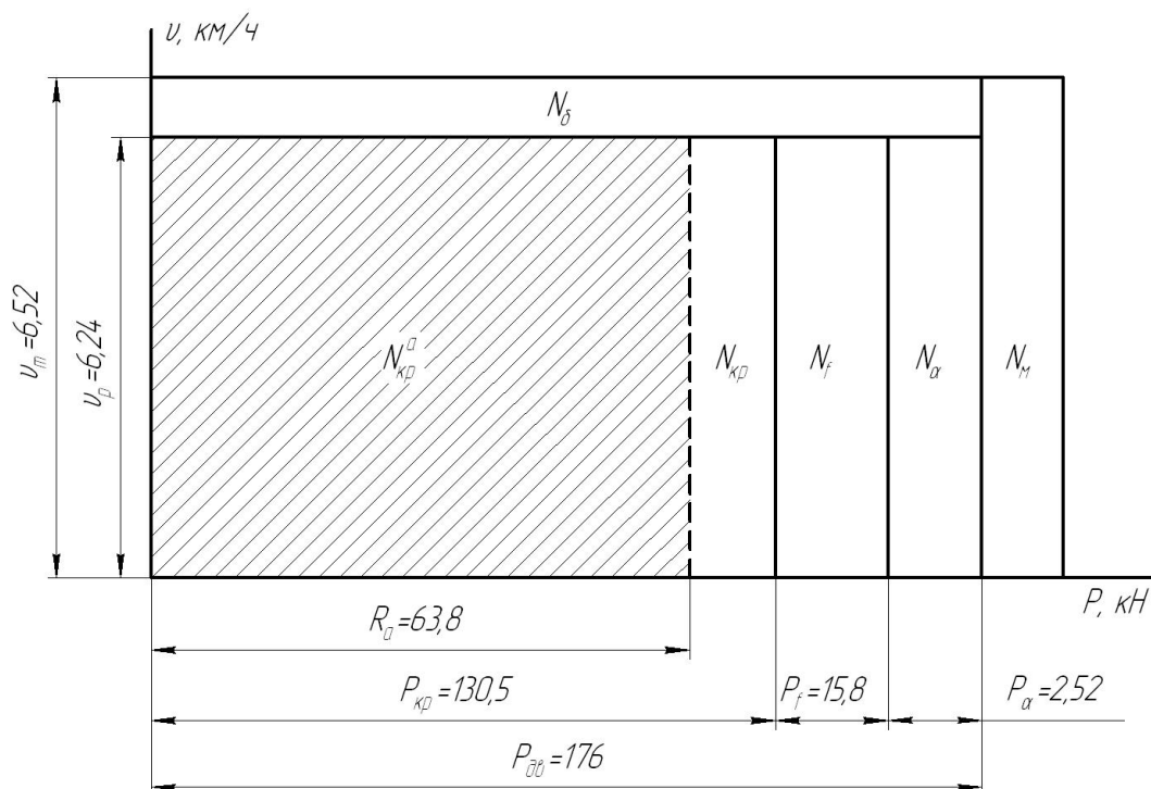
Рисунок 2 – График баланса мощности
