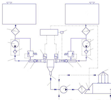
Рисунок 1. Двухтопливная система питания дизеля: расшифровка позиций
